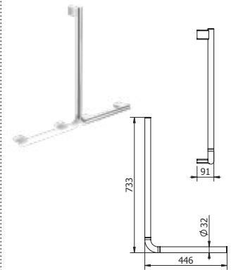
DIANA C100 Haltegriff verchromt, 90°, links und rechts montierbar, Einhängeklappsitz möglich, 446 x 733 mm, (DI617020500) 407,- €
