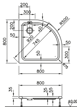
DIANA S100-Neu Acryl-Viertelkreis-Brausewanne superflach, Weiß, 800 x 800 mm, Tiefe 35 mm, Ablaufloch 90 mm, (DI224251001) 369,- €
