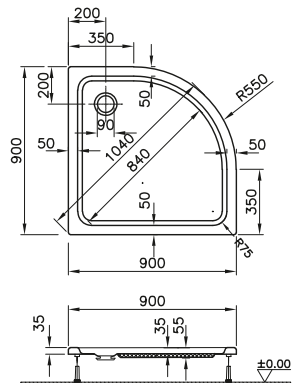
DIANA S100-Neu Acryl-Viertelkreis-Brausewanne superflach, Weiß, 900 x 900 mm, Tiefe 35 mm, Ablaufloch 90 mm, (DI224252001) 378,- €
