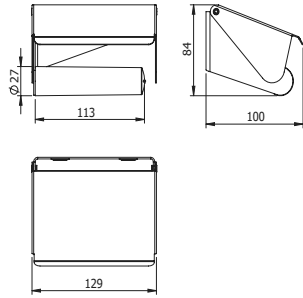
DIANA O100 Haubenpapierhalter verchromt, mit lichtgrauer Rolle, (DI601606500) 42,30 €
