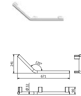
DIANA C100 Winkelgriff verchromt, 135°, Ausführung links, (DI617071500) 296,- €
